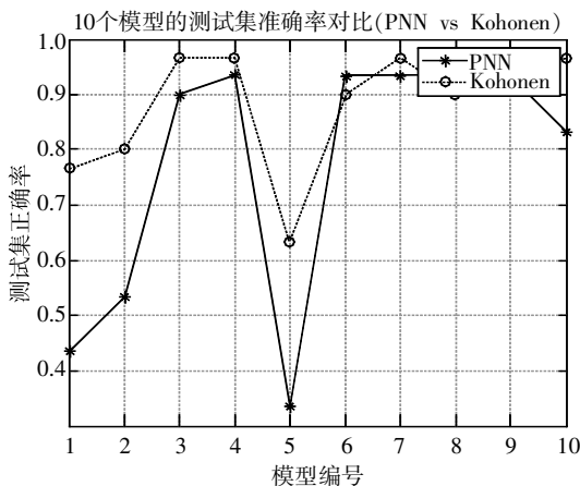
图9 测试准确率对比图
